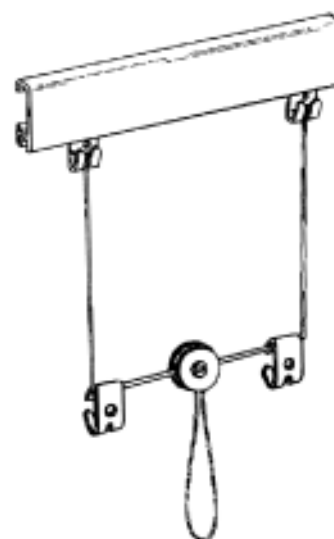
Komplet za držanje slike 7
