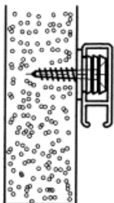
Zidna montaža sa podloškama AL3432K
