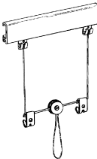
Sastavljanje kompleta za držanje slike - komplet 7
