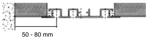
Stropna montaža u spuštenu strop
