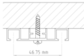
Stropna montaža AL 360
