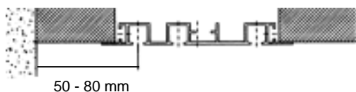
Stropna montaža u spuštenu strop sa profilnim nosačem AL2535
