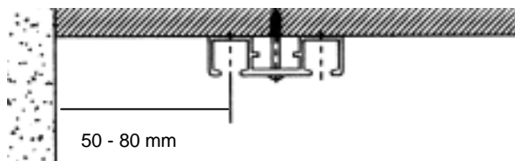
Stropna montaža AL 350
