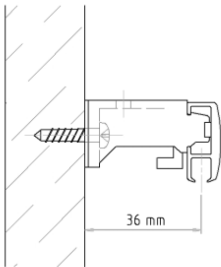
Zidna montaža 1 vod. sa nosačem AL3420K
