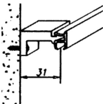
Zidna montaža 1 vod. sa nosačem AL3440K
