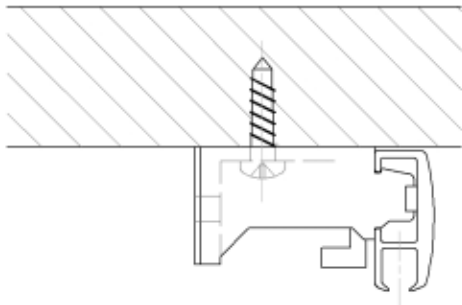
Stropna montaža 1 vod. sa nosačem AL3420K
