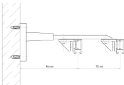
Zidna montaža 2 vod sa nosačima AL2511K i AL7354K
