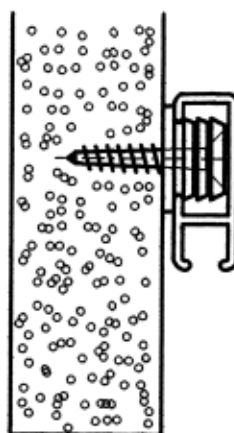
Zidna montaža sa podloškom AL3432K
