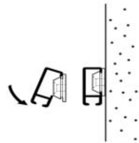
Zidna montaža sa podloškama AL7351K
