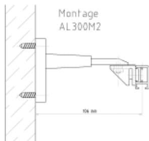
Zidna montaža 1 vod sa nosačima AL2525K i AL7354K
