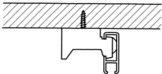
Stropna montaža sa nosačem AL3420K
