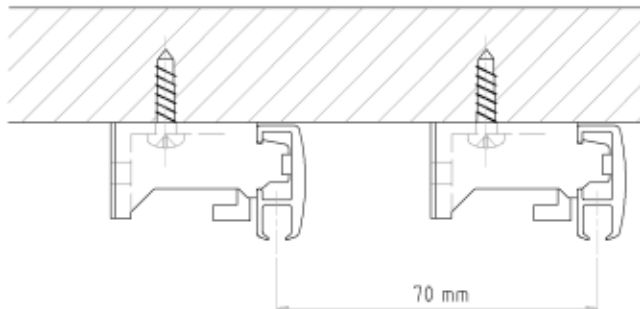
Stropna montaža 2 vod. sa nosačem AL3420K
