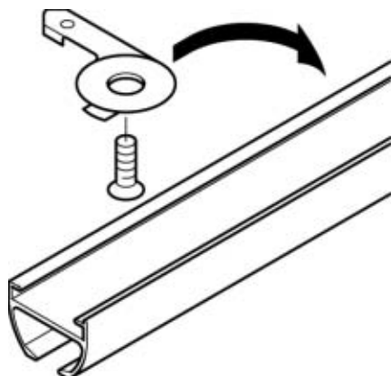
Stropna montaža sa nosačem AL7607K
