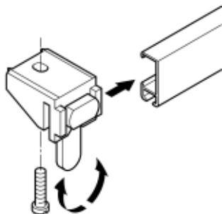
Stropna montaža sa nosačem AL7354K
