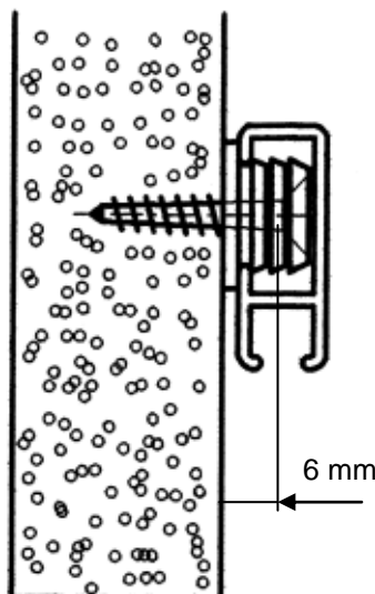
Zidna montaža 1 vod. sa podloškomo za zidnu montažu AL3432K
