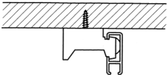
Stropna montaža 1 vod. sa nosačem AL3420K
