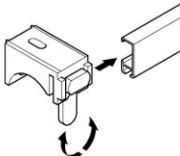
Zidna montaža sa nosačem AL7352K
